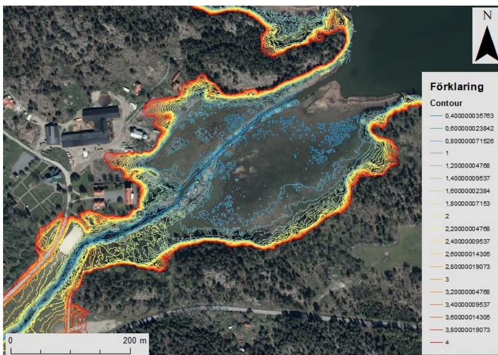
Figur 19. Höjdkurvor vid mynning av Jonsbergsån. Angivna nivåer i beskrivningen är meter över havet angett i systemet RH2000.
