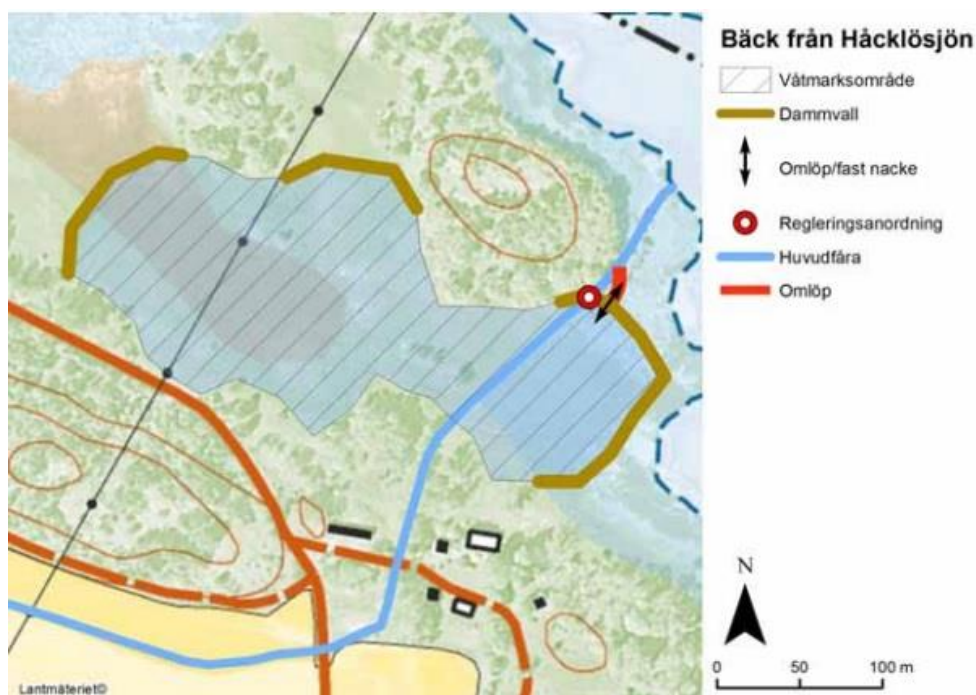
Figur 16. Principskiss för den potentiella våtmarken i mynningsområdet.
