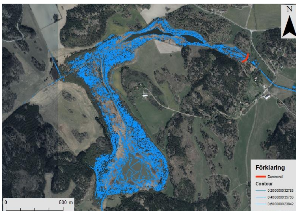
Figur 50. Laserskannade höjddata över Rönöån, Övre och nedre sundet. Angivna nivåer i beskrivningen är meter över havet angett i systemet RH2000.
